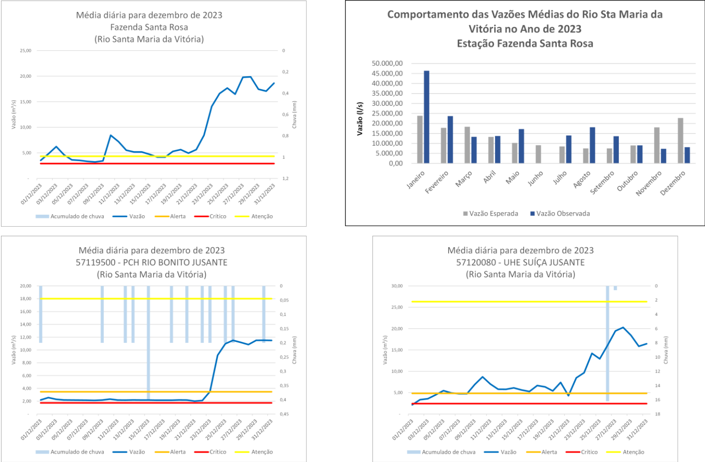
Figura 5: Vazões médias diárias (Dez/2023) e Comportamento das vazões médias - Estações Hidrológicas Indicadoras. Fonte: Cohip/Agerh.
