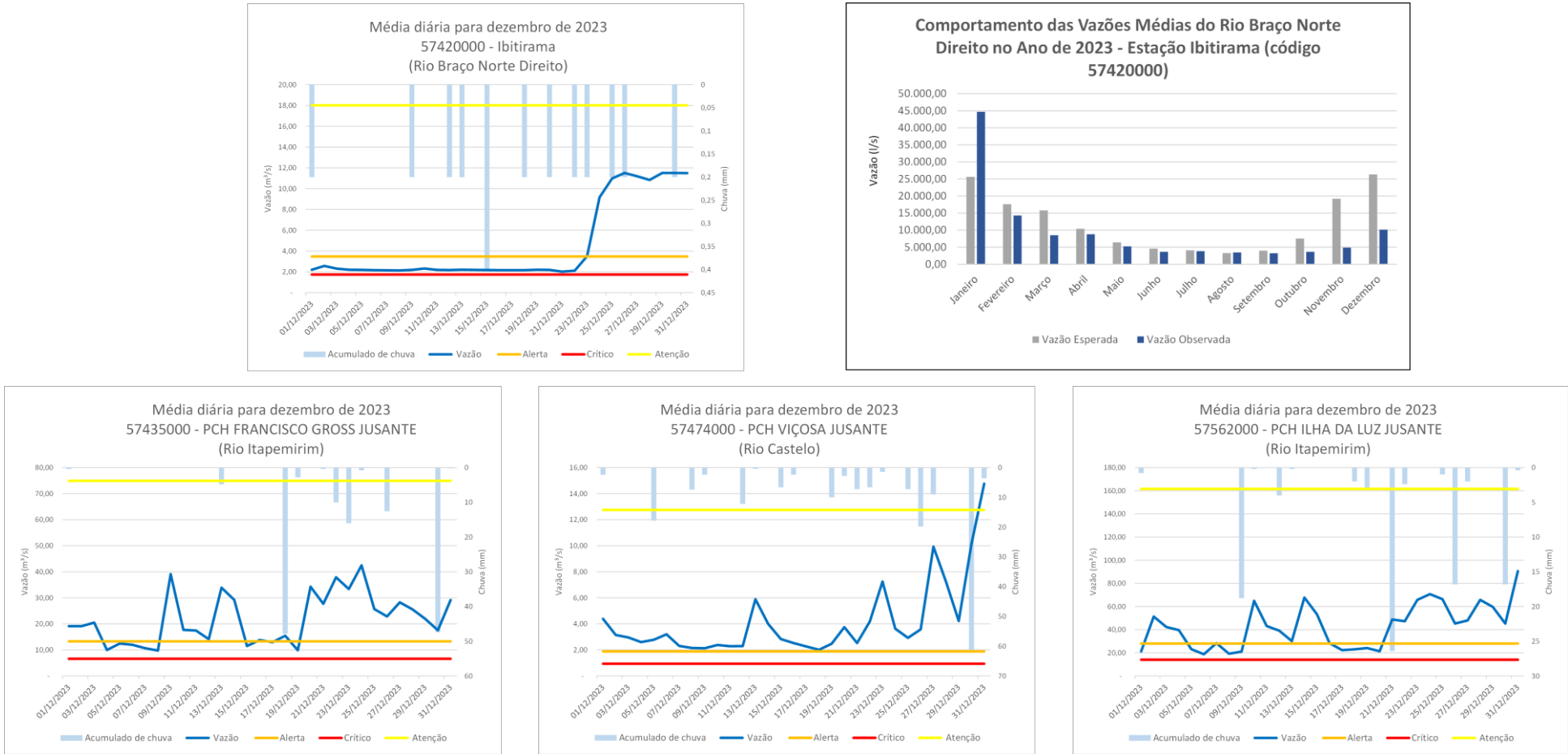
Figura 5: Vazões médias diárias (Dez/2023) e Comportamento das vazões médias - Estações Hidrológicas Indicadoras. Fonte: Cohip/Agerh.
