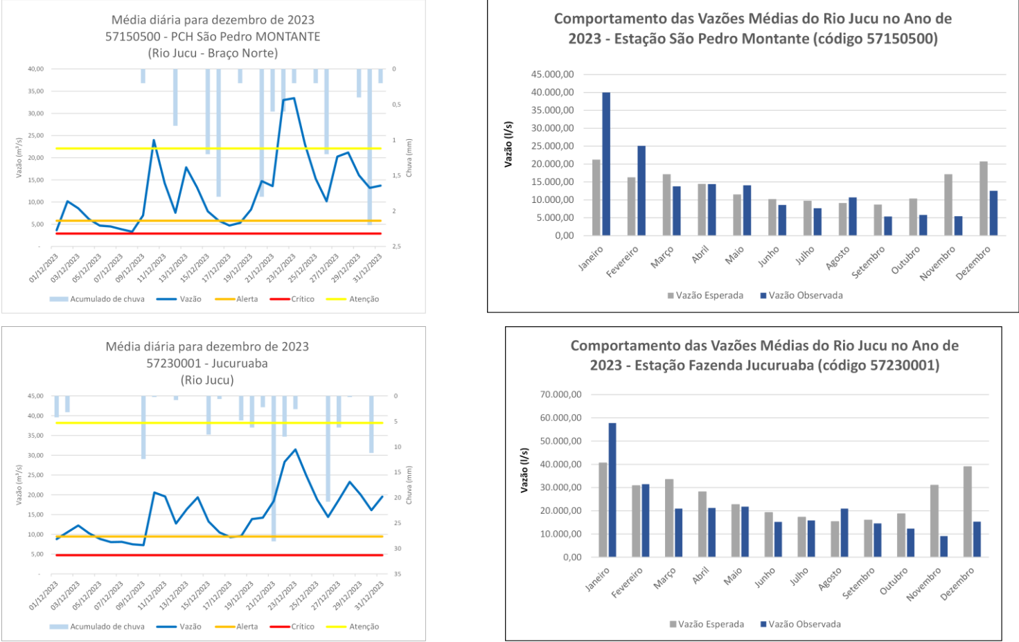
Figura 5: Vazões médias diárias (Dez/2023) e Comportamento das vazões médias - Estações Hidrológicas Indicadoras. Fonte: Cohip/Agerh.
