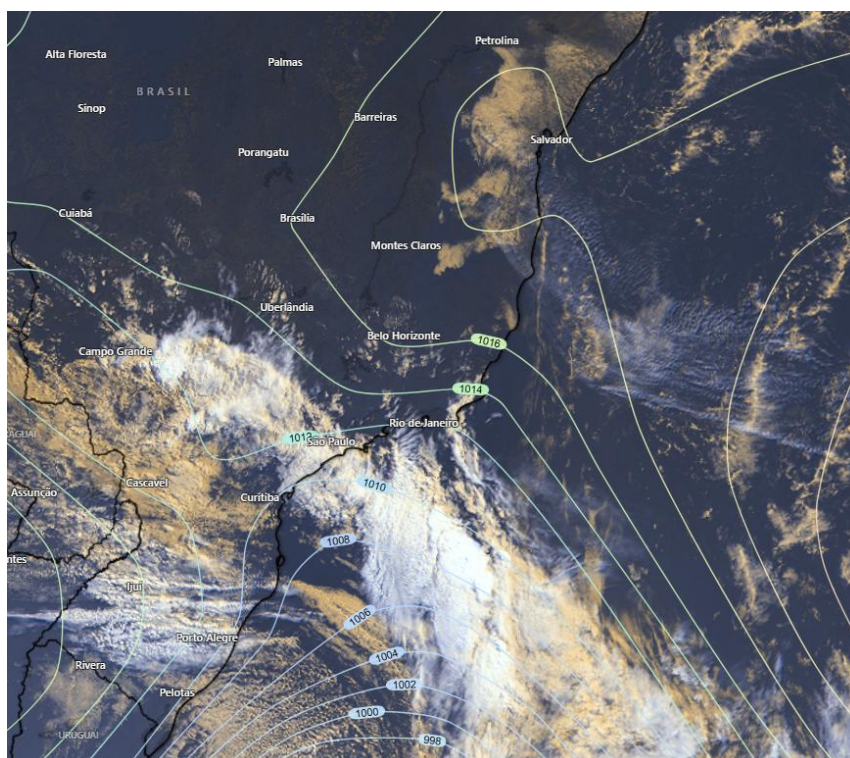
Figura 1 – Imagem do satélite GOES-19 (canal visível) e isóbaras às ~10:00 UTC de 07/08/2026.
