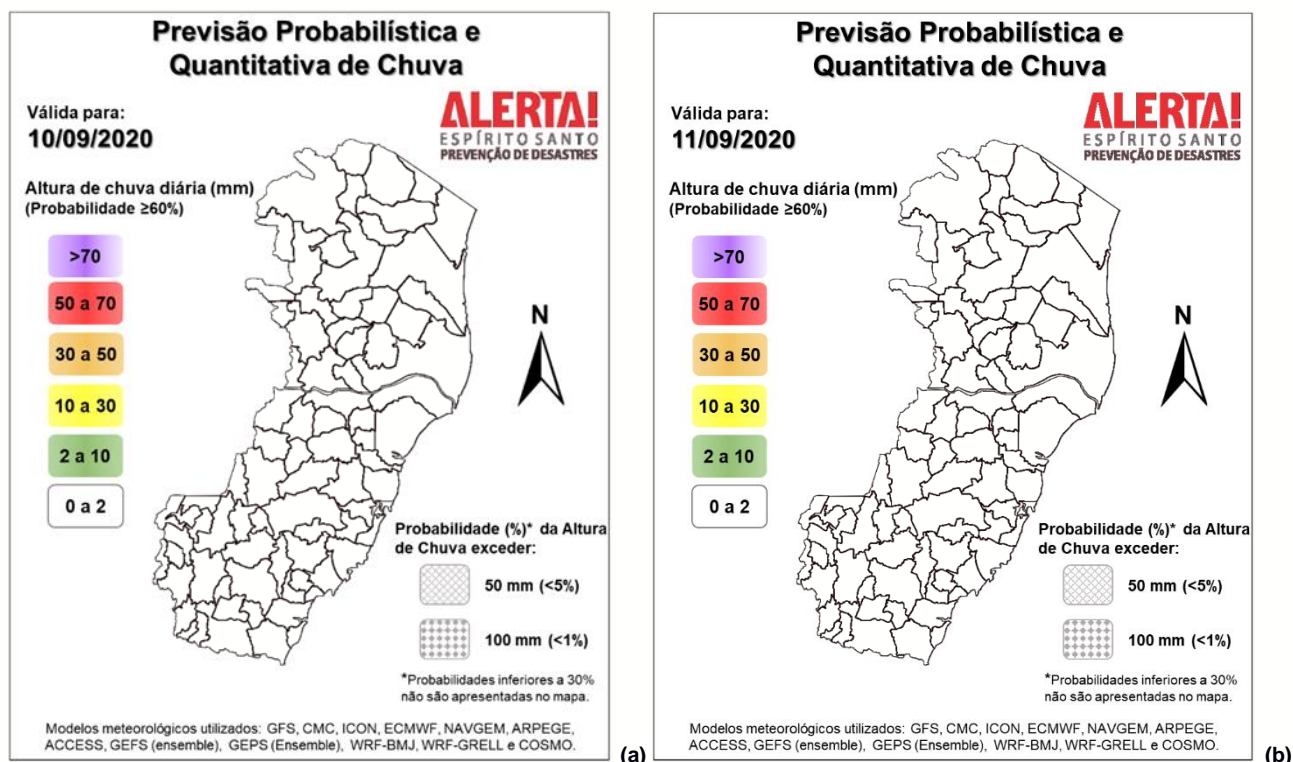
Figura 2 – Previsão quantitativa (mm/24h) e probabilística (%) de precipitação para 10 (a) e 11/09/2020 (b).
