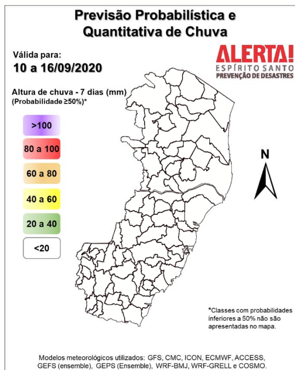
Figura 3 – Previsão quantitativa (mm) de precipitação acumulada para o período de 10 a 16/09/2020.
